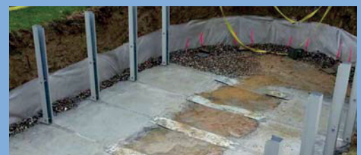
Spezielles Ovalbecken: Einbetonieren der seitlichen Stützen
