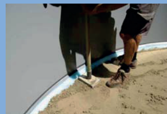
Schlemmsand verdichten
