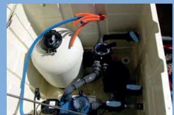
Montage der Filtertechnik.
