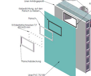
Einbauteile abflanschen
